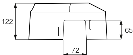
Vue Dessous
