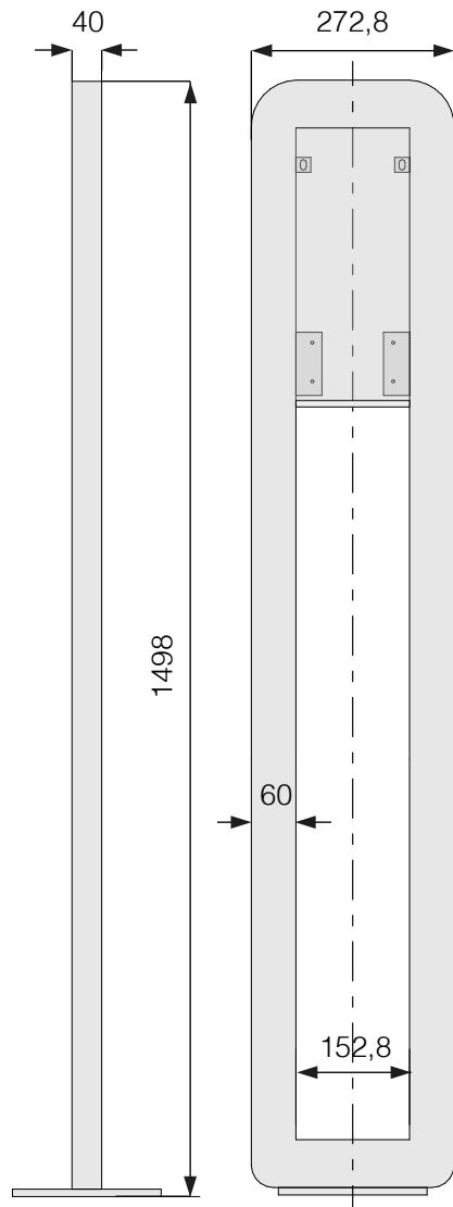
Vue latérale
